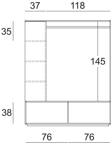
RBWAP8 isola centro stanza middle unit
